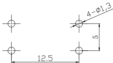
PCB. 焊接图
