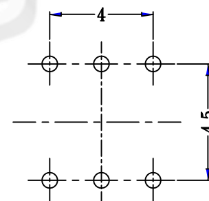
P.C.B. LAYOUT
